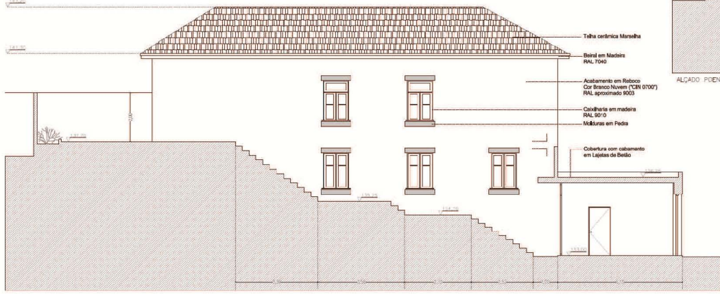
ALÇADO NASCENTE
