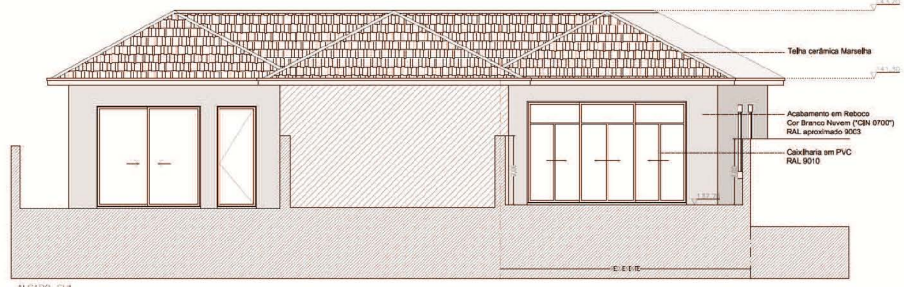
ALÇADO SUL
