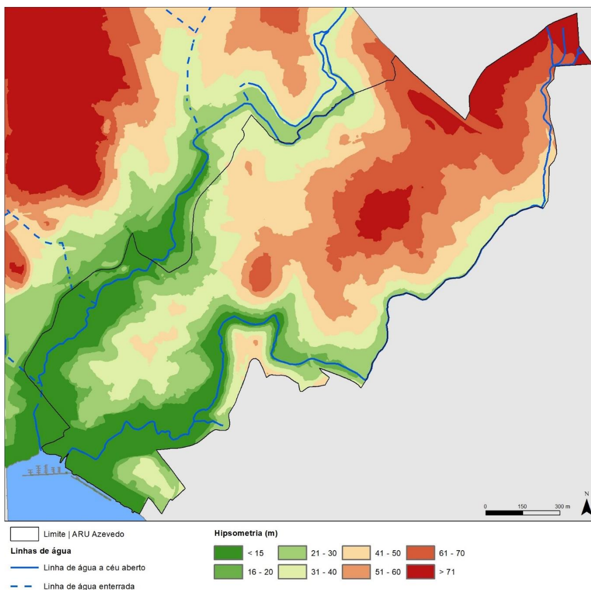
Figura 32. Hipsometria da ARU de Azevedo e da sua envolvente
