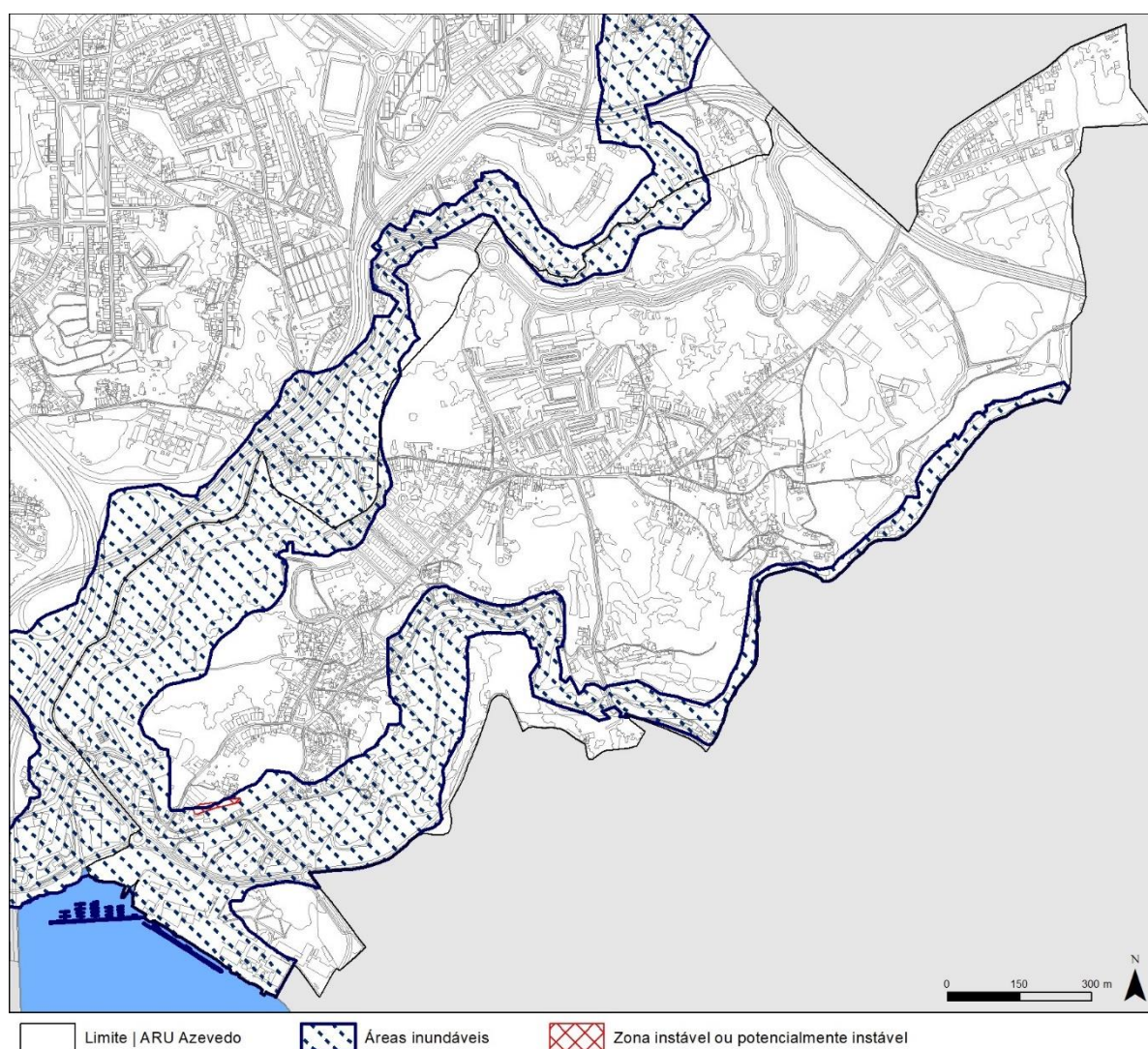
Figura 33. Planta de Ordenamento – Carta de Riscos Naturais (PDM 2021)
