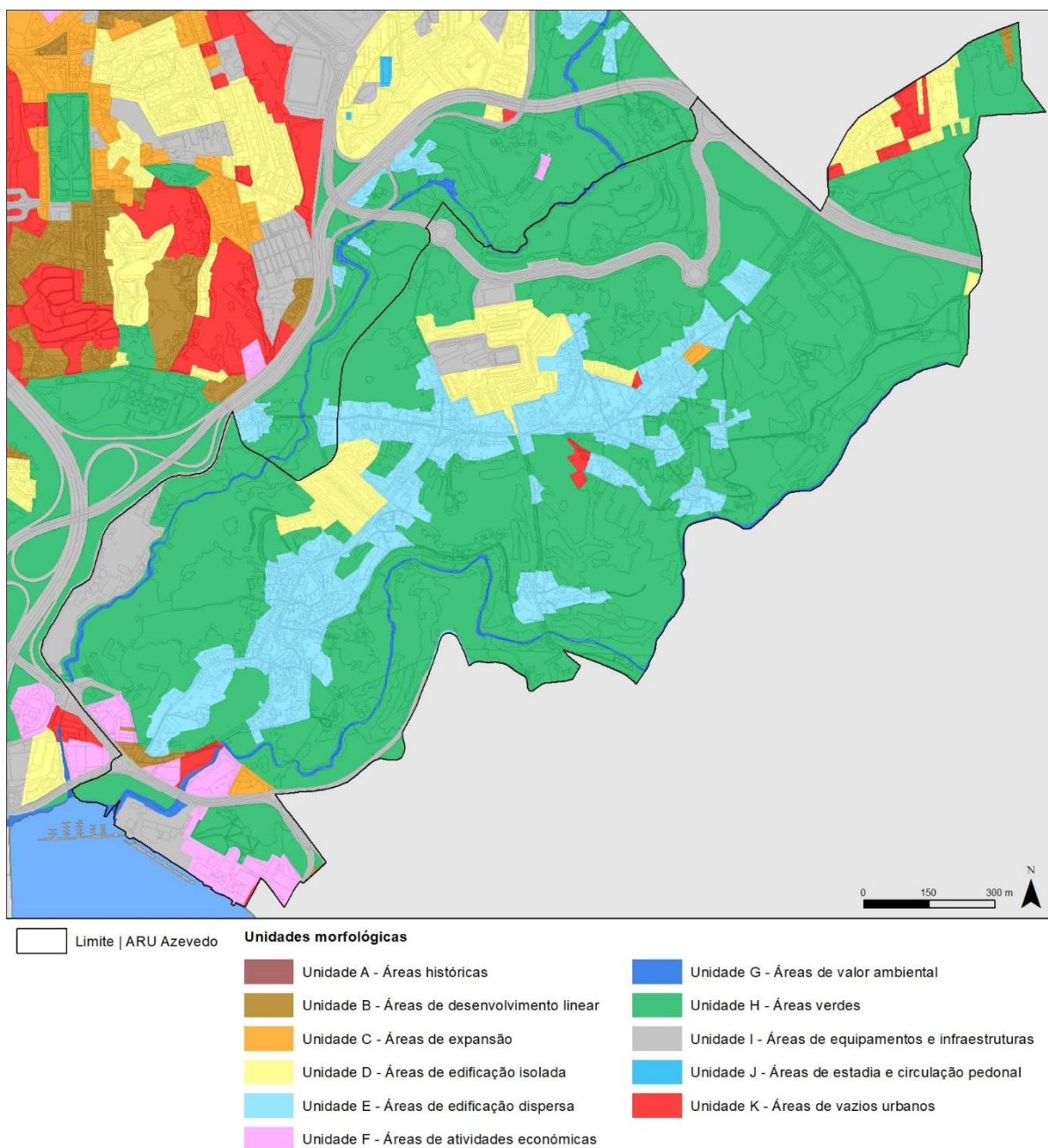
Figura 36. Ocupação do solo da ARU de Azevedo e da sua envolvente
