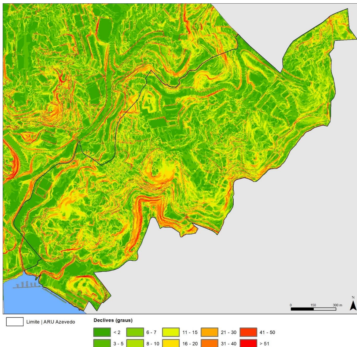
Figura 34. Declives da ARU de Azevedo e da sua envolvente
